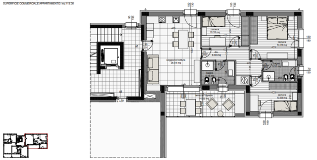
EDIFICIO A - PIANO SECONDO - APPARTAMENTO A7
